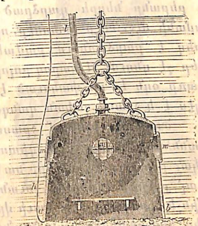
Նկ. 2. Ջրասուզական զանգակ: m, m—պատուհանները. l—օդի խողովակը. h—հնչակի շւանը:
