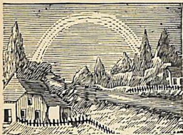
Պատկ. 7. — Ծիածան
