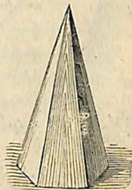
Պատկ. 49. Կոն
