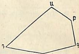
Պատկ. 22. Բազմանկիւն
