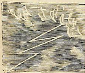
Պատկ. 5. — Կայծակ
