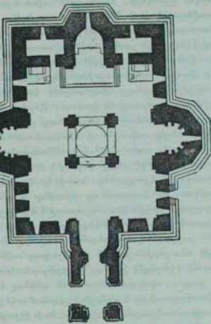
Յաստակացի իշխան . — Plan de la Cathédrale.
