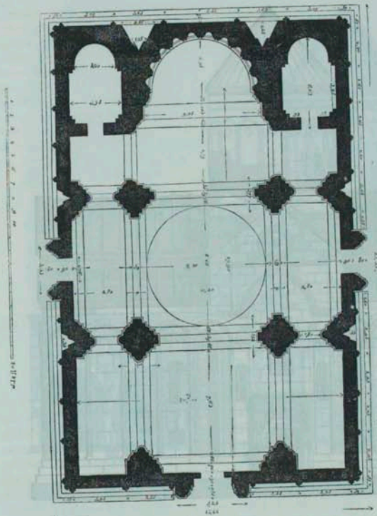
Յատակագիծ կարող. Սևայ. — Plan de la Cathedrale.
