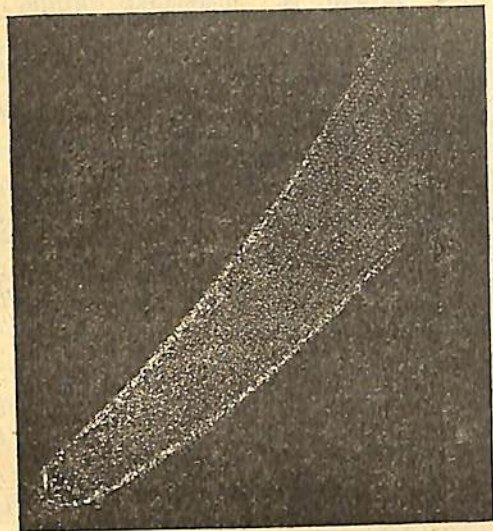
Պատկ. 5. — 1811ի Գիսաւորը
