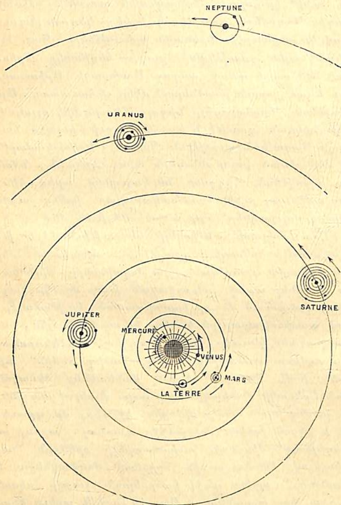
Պատկ. 2. — Արեգակնային դրութիւն
