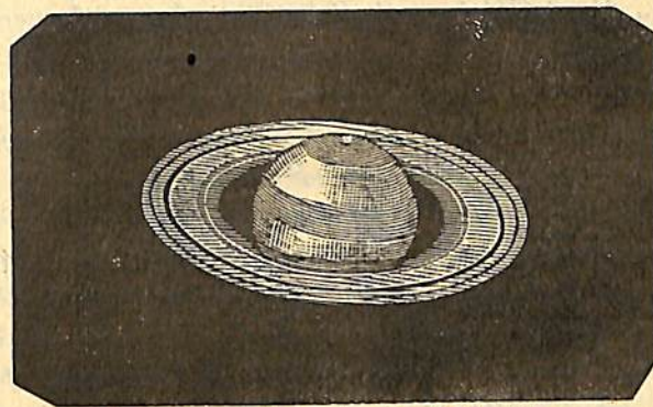
Պատկ 4. — Նրեւակ ու իր մասնակները
