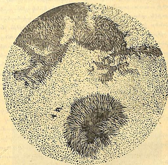
Պատկ. 3. — Արեւական բիծերը
