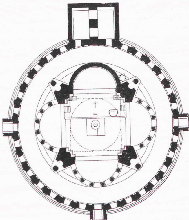
Յասակագիծ Զուարթնոց եկեղեցւոյ
